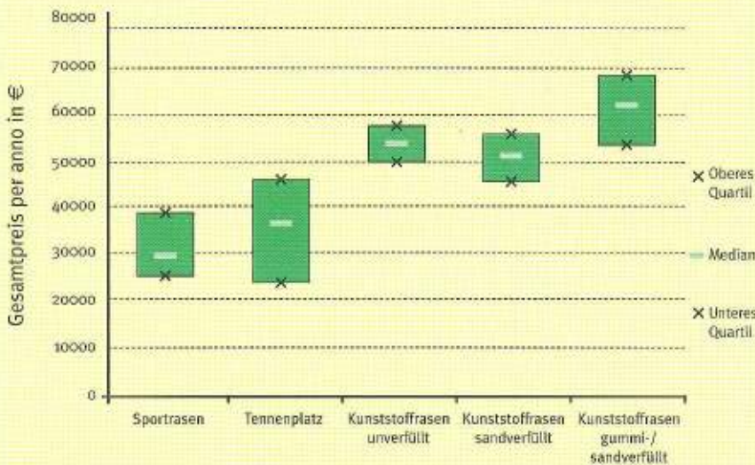
Abb. 5: Lebenszykluskosten bei einer dreißigjährigen Nutzung*
