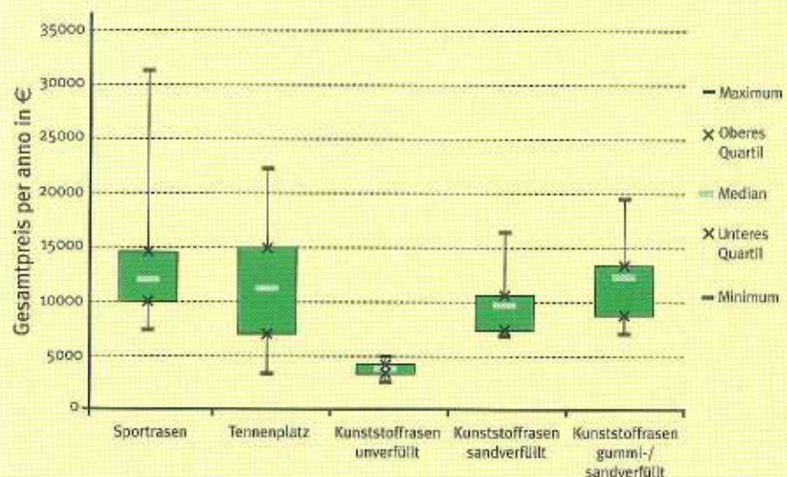
Abb. 4: Pflegekosten für verschiedene Belagsarten
